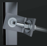
斜拉安装
