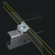
侧压块安装
