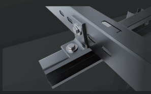
檩条安装
