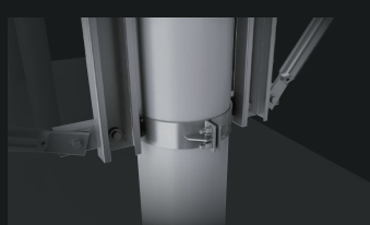
抱箍安装
